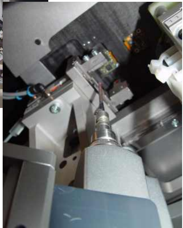
Station 3 Blick von unten auf Prüfling und Schrauber
