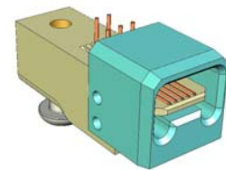
USB plug mini Type B with center unit
